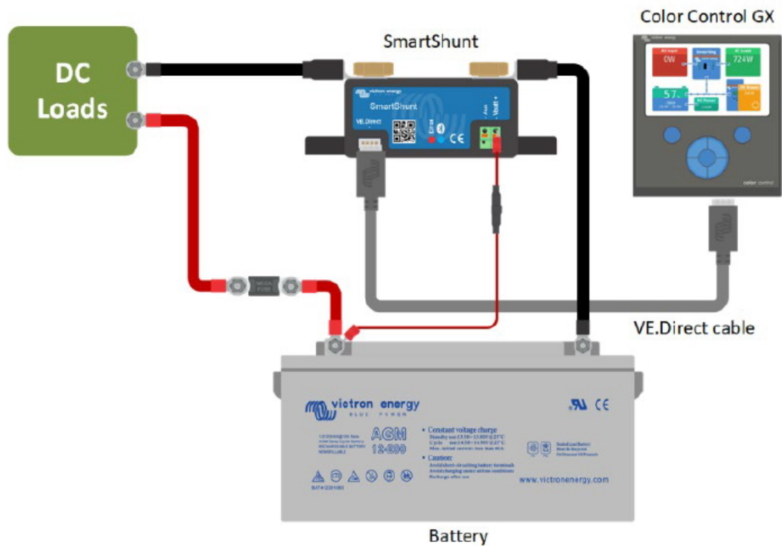
Schéma zapojení se zařízením GX:
