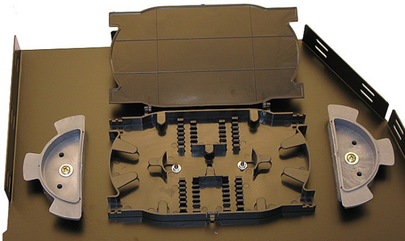
Přívod kabelu
